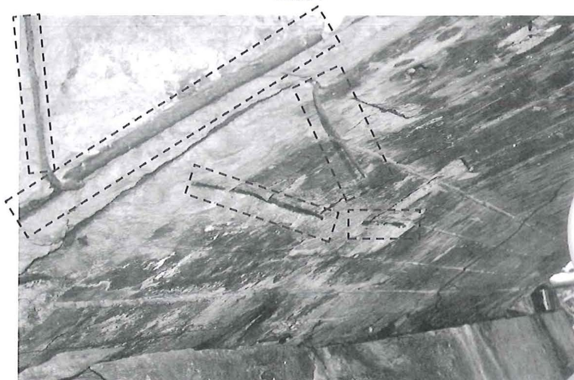
Figura 4 – Perda de cobrimento do concreto com armadura exposta em estado avançado de corrosão e perda de seção, identificando perda de funcionalidade da mesma
