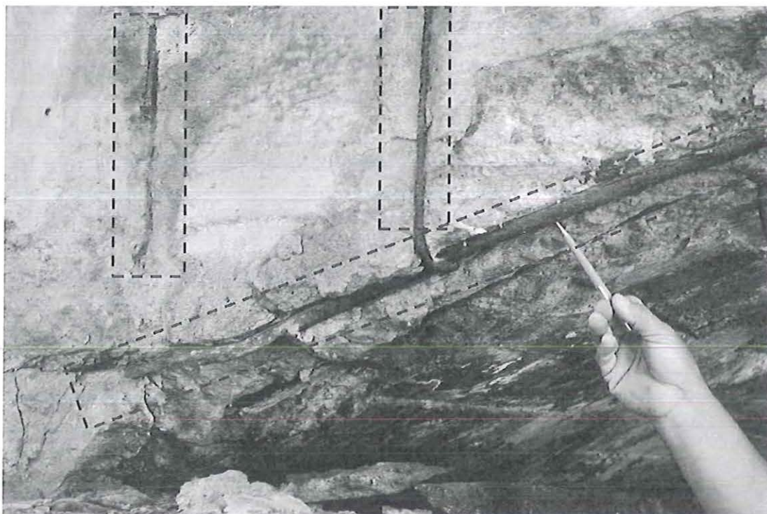
Figura 3 – Perda de cobrimento do concreto e armadura exposta em avançado estado de corrosão na estrutura da ponte, no apoio situado no lado esquerdo da estrutura conforme
