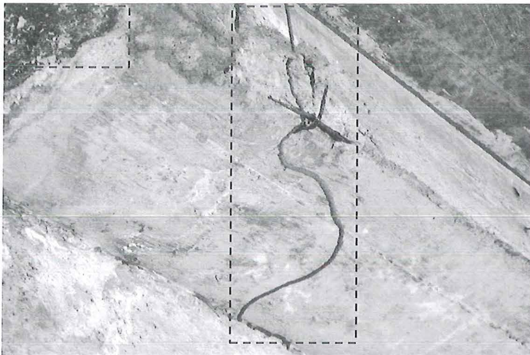
Figura 7 – Presença de cupim, armadura exposta e lixiviação na estrutura da ponte
